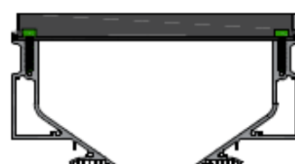
Перфорация (ПФ)
