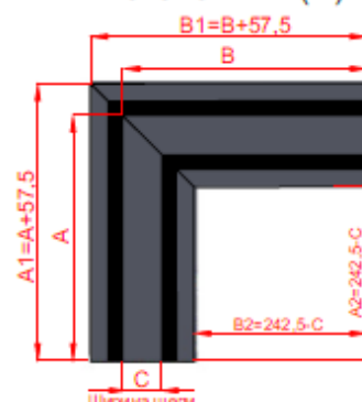
Потолочный (П)
