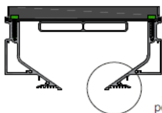
Дефлектор (ДФ-Фикс)
